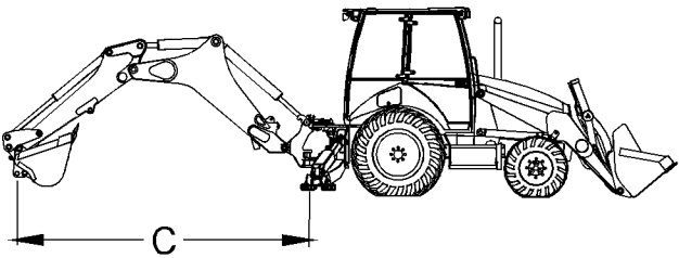
Ilustración 55 g01327477 Radio del punto de levantamiento (A)
