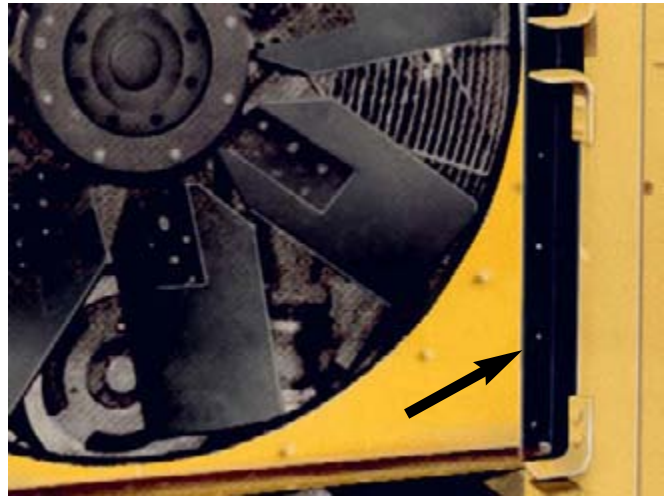
Fig. 61: Radiator Baffle.
