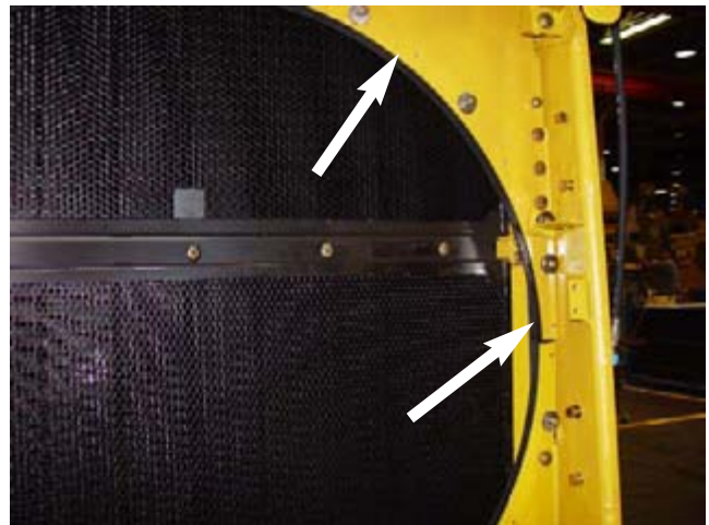
Fig. 62: Fan shroud.
